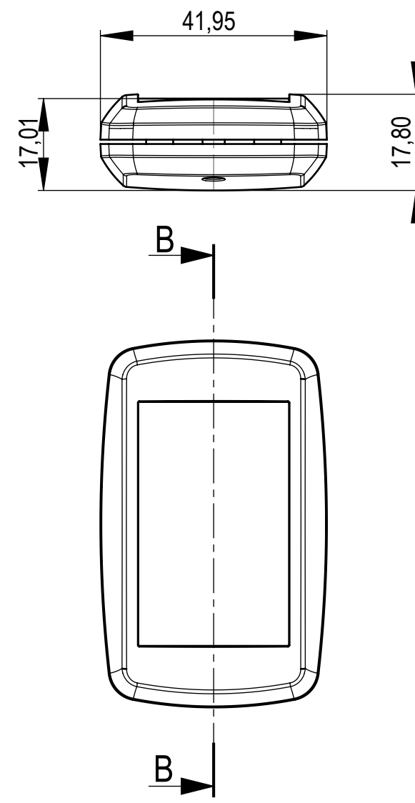
Oberteil mit Vertiefung top part with recessed area
