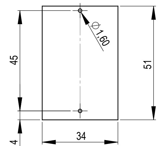
Platine UT P C B
