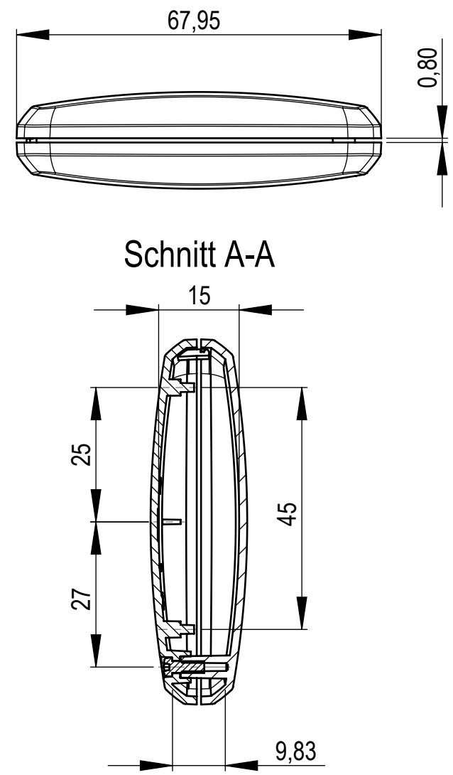
mit 1 Öse with 1 strap loop
