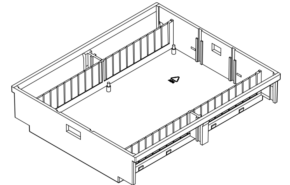
Platine Oberteil PCB top
